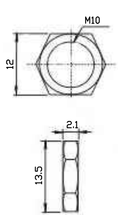
HEX NUT
