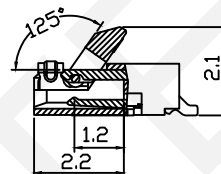
SECTION A-A SCALE 2:1
