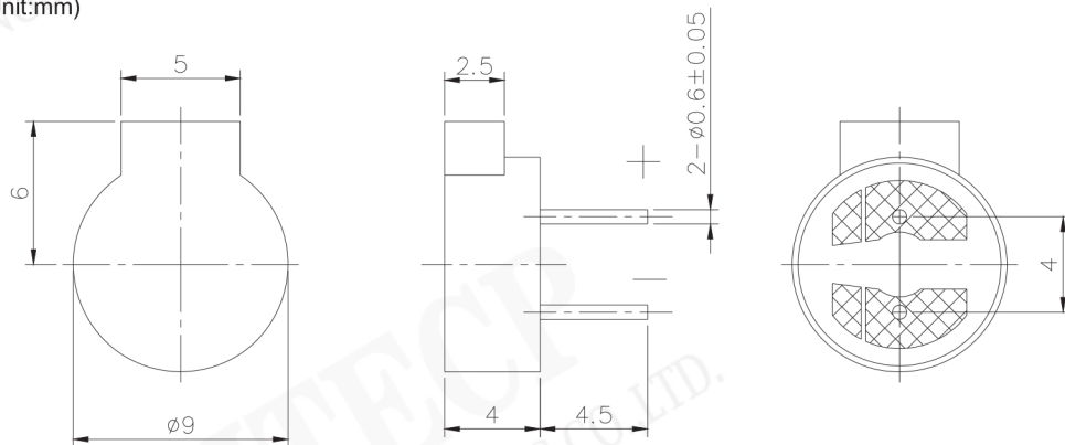
Dimensions (Unit:mm)
